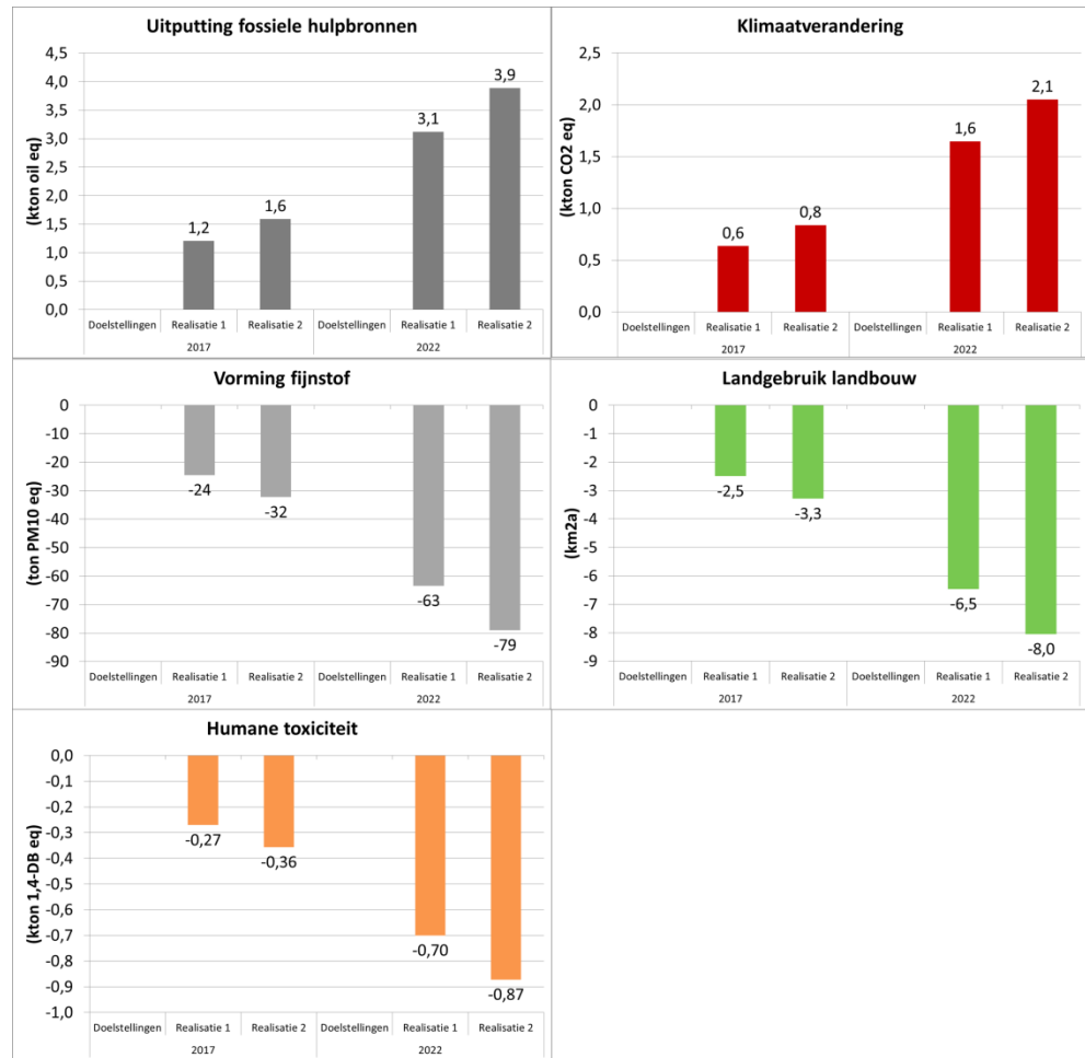
Figuur 41 Gekarakteriseerde waarden voor de vijf aan de endpoint single score meest bijdragende effectcategorieën voor het doelstellingscenario en realisatiescenario 1 en 2 voor de jaren 2017 en 2022 ten opzichte van 2012.
