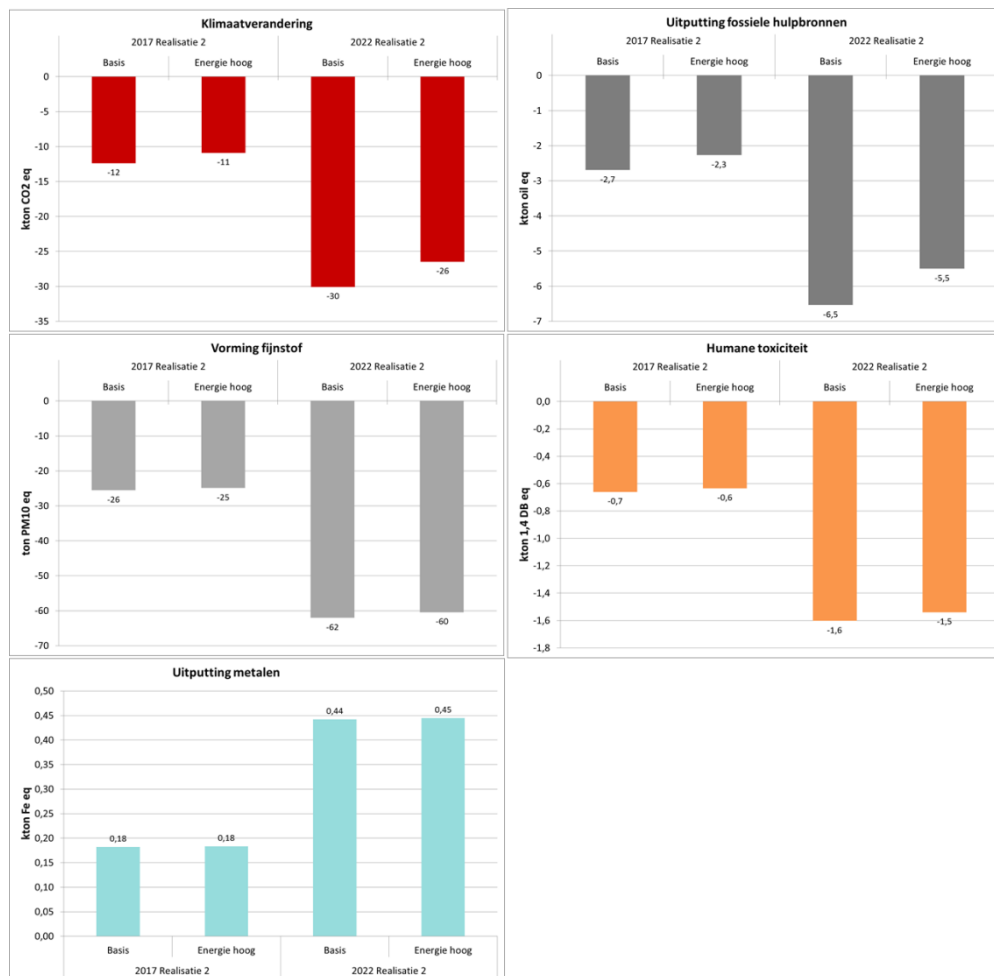
Figuur 54 Gevoelighedsanalyse voor de vijf meest bijdragende effectcategorieën aan de endpoint single score voor de toename van het elektriciteitsgebruik bij de aluminiumsortering voor de additionele aluminium recycling 'Energie hoog'.
