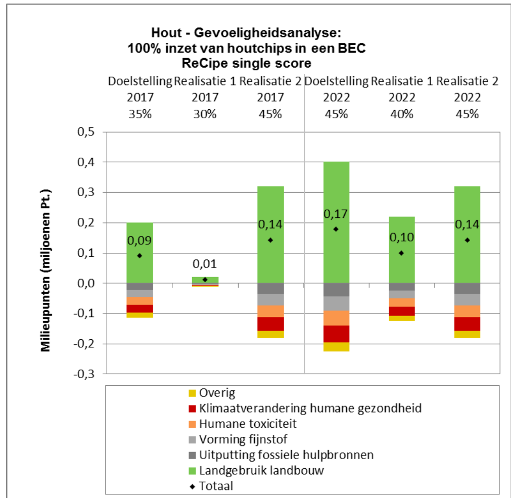
Figuur 37 Hout, gevoeligheidsanalyse: 100% compensatie door chips bij verbranding.
